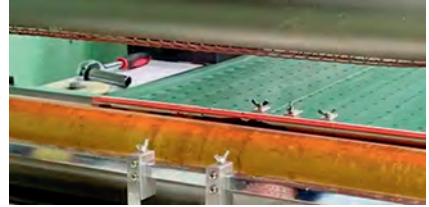
Каширування
